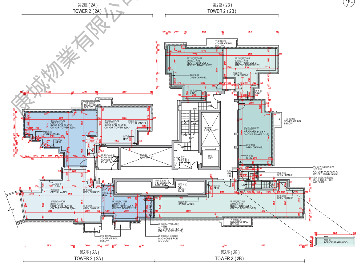
Tower 2(2A) & Tower 2(2B) Roof Floor Plan 第2座(2A)及第2座(2B)天台樓面平面圖
